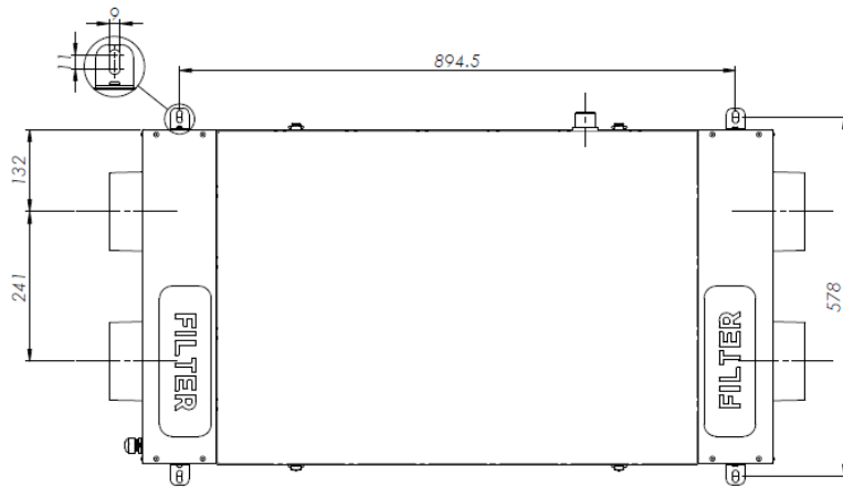
OXYGEN X-Air C180 kairinė versija
