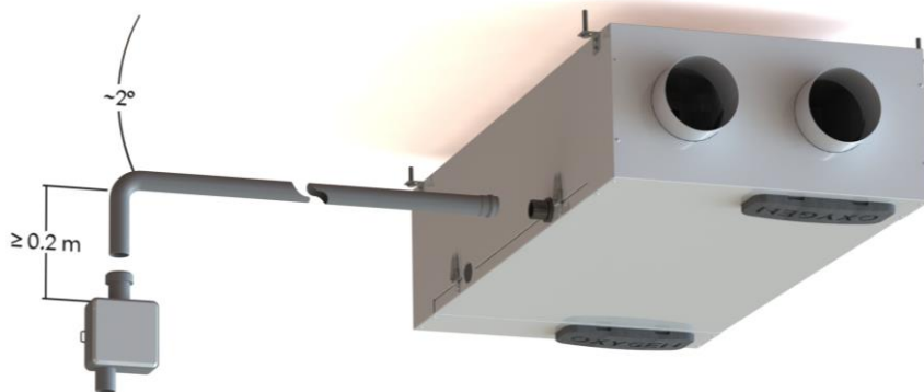
Pav. 7. Kondensato surinkimo latako prijungimas
