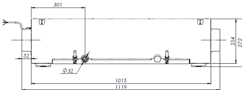
Pav. 1. Vėdinimo įrenginio matmenys
