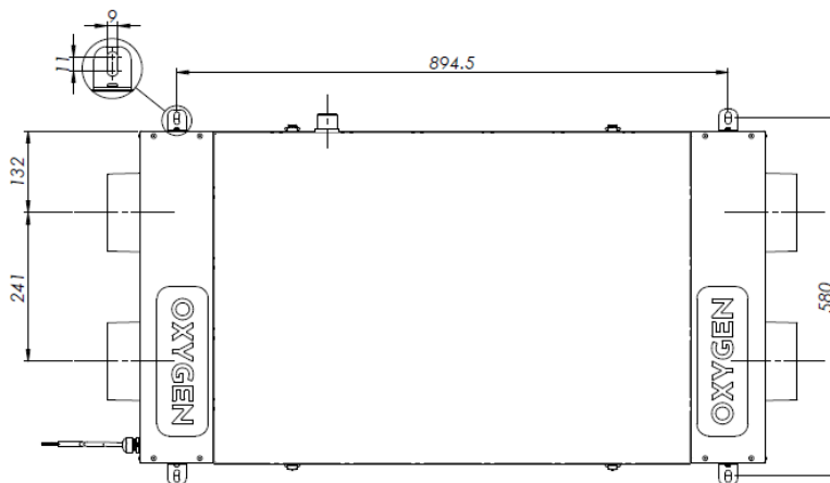
OXYGEN X-Air C180 dešininė versija
