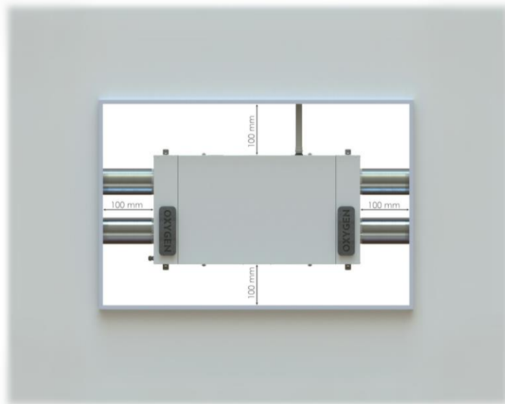
Pav. 5. Priežiūros bei aptarnavimo liukas
