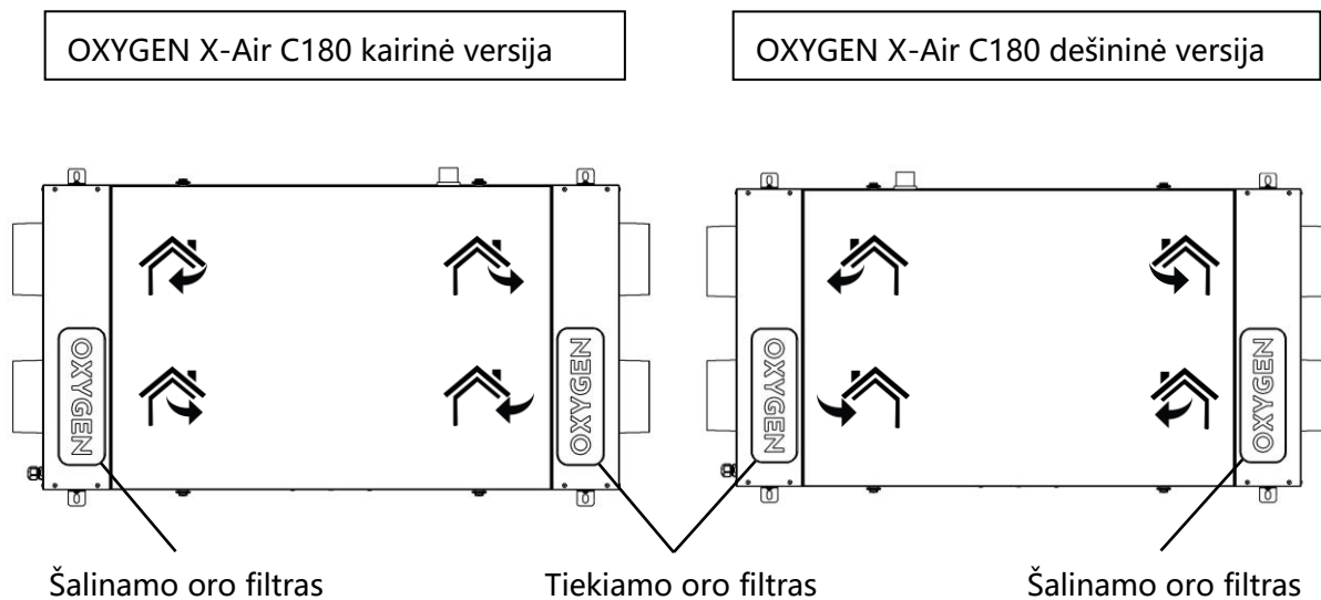
Pav. 13. Vėdinimo įrenginio filtrai
