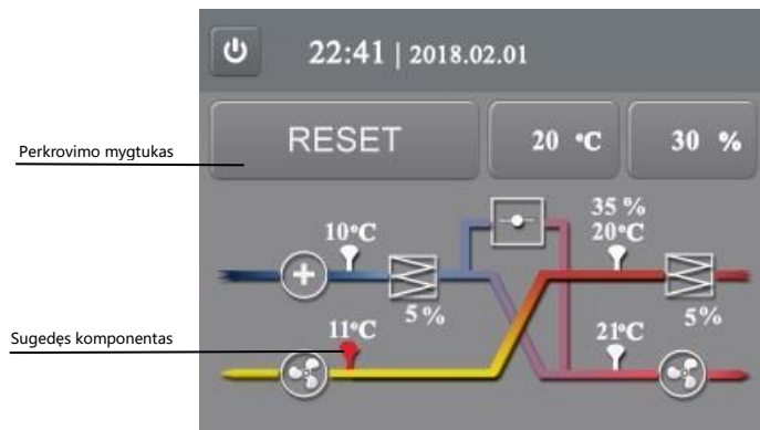
Pav. 30. Vėdinimo įrenginio gedimo indikacija
