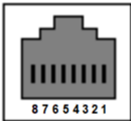
Pav. 10. Funkcijų jungties kontaktai
