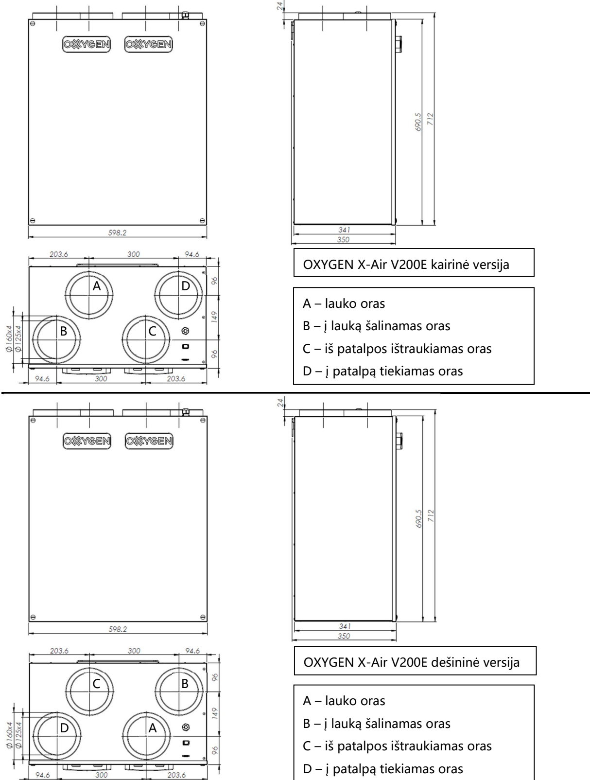
Pav. 1. Vėdinimo įrenginio matmenys
