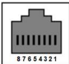
Pav. 8. Funkcijų jungties kontaktai
