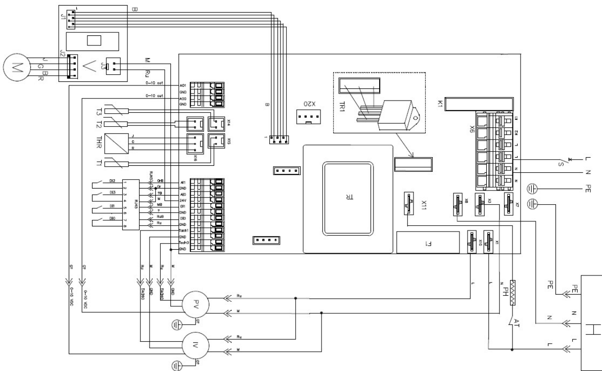
Pav. 10. Vėdinimo įrenginio valdymo plokštės elektrinio jungimo schema
