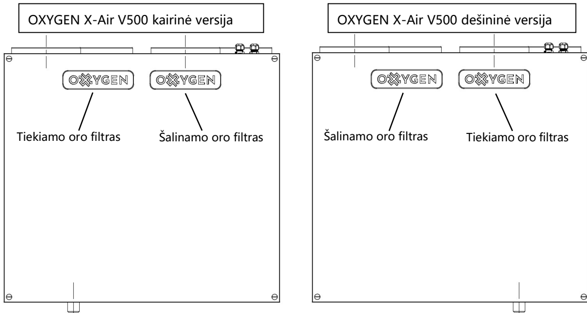
Pav. 28. Vėdinimo įrenginio filtrai
